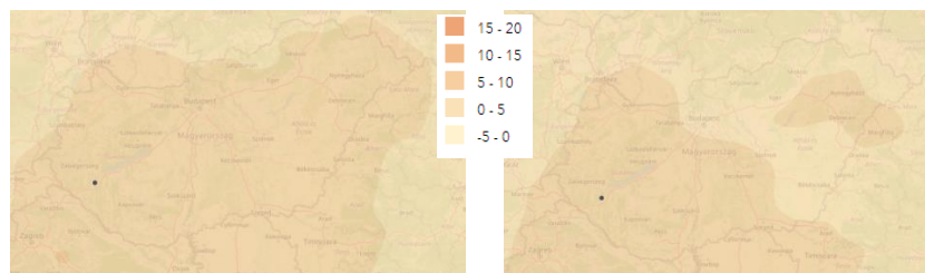
1.20-1. ábra: Hőségriadós napok éves átlagos számának változása Magyarországon a 2021-2050 időszakra, az 1970-2000 közötti referenciaidőszakhoz viszonyítva, nap
