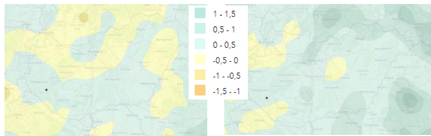
1.20-2. ábra: 30 mm-t meghaladó csapadékösszegű napok átlagos éves számának várható változása Magyarországon a 2021-2050 időszakra, az 1970-2000 közötti referenciaidőszakhoz viszonyítva (nap)
