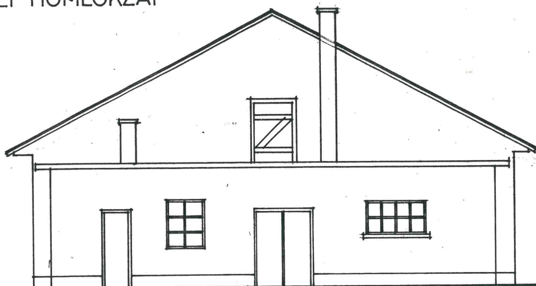
DÉLI HOMLOKZAT
